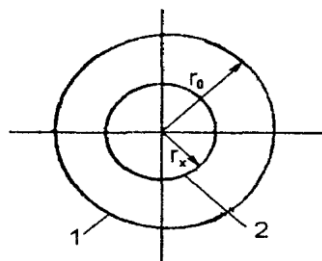
Рисунок Б.1. Зона защиты одиночного стержневого молниеотвода высотой до 150 м: 1 - граница зоны защиты на уровне земли; 2 - то же на высоте h_x .
