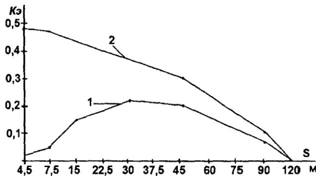
Рисунок А.1 - Коэффициенты экранирования для одностороннего экранирующего объекта высотой, равной h_{\text{вл}}/2 (1) и h_{\text{вл}} (2), при различных расстояниях S от ВЛ. Высота ВЛ h_{\text{вл}} = 9-15 м
