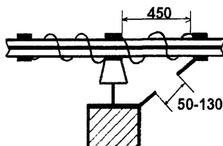
Рисунок Ж.5 - Искровые промежутки на опоре с металлической траверсой для защиты ВЛЗ 6-10 кВ от дуговых повреждений при расстоянии между проводами на опоре более 0,6 м
