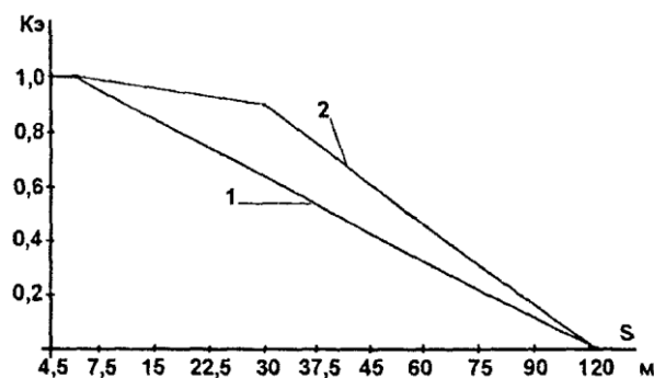
Рисунок А.2 - Коэффициенты экранирования для объектов высотой (1,5-2)h_{\text{вл}} одностороннего (1) и двухстороннего (2), при различных расстояниях S от ВЛ. Высота ВЛ h_{\text{вл}} = 9-15 м
