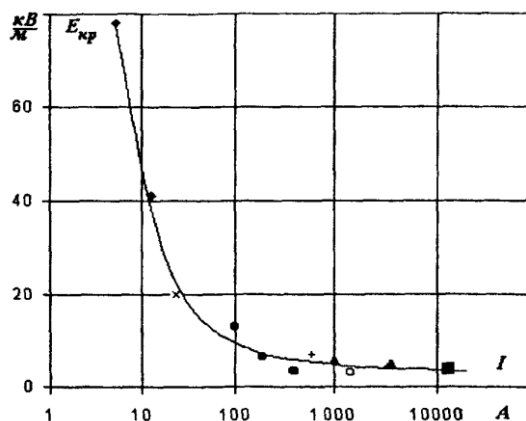
Рисунок Г.4 - Зависимость критического градиента перехода импульсного перекрытия в дугу от сопровождающего тока
