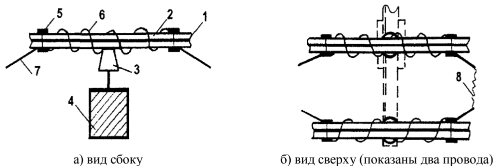
Рисунок Ж.4 - Защита ВЛЗ 6-10 кВ с двухсторонним питанием от дуговых повреждений с использованием "защитных рогов":
