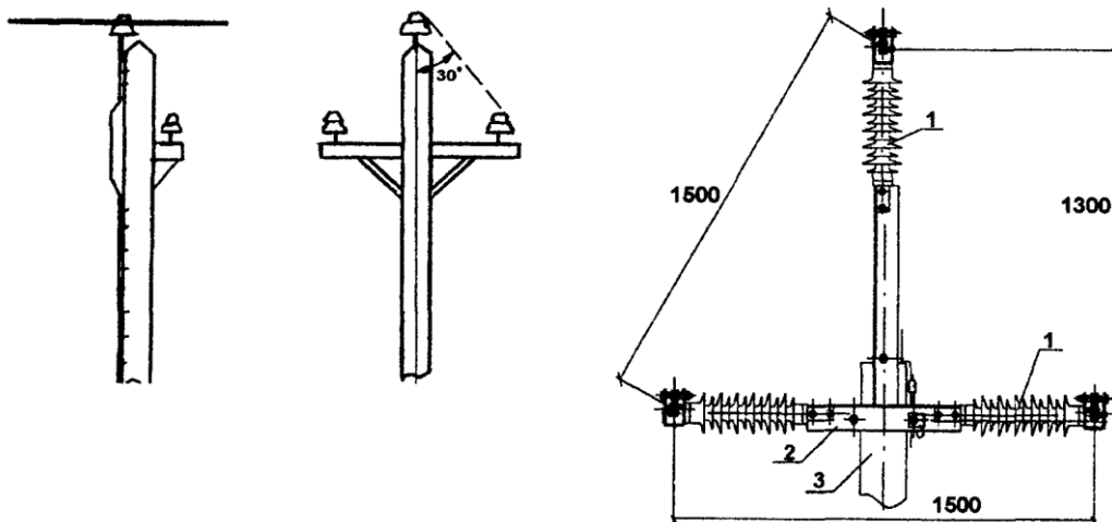
Рисунок Ж.2 - Деревянные или железобетонные опоры ВЛ 10 кВ с изоляционной траверсой и защитным проводом
